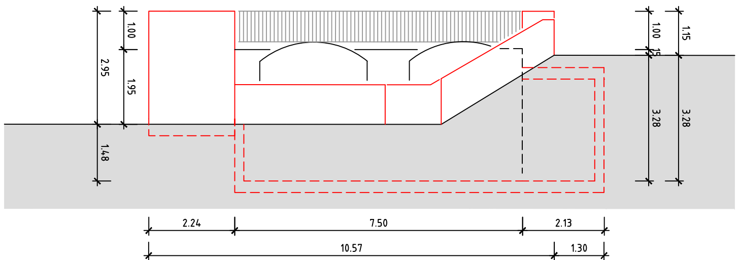
Ansicht Ost
